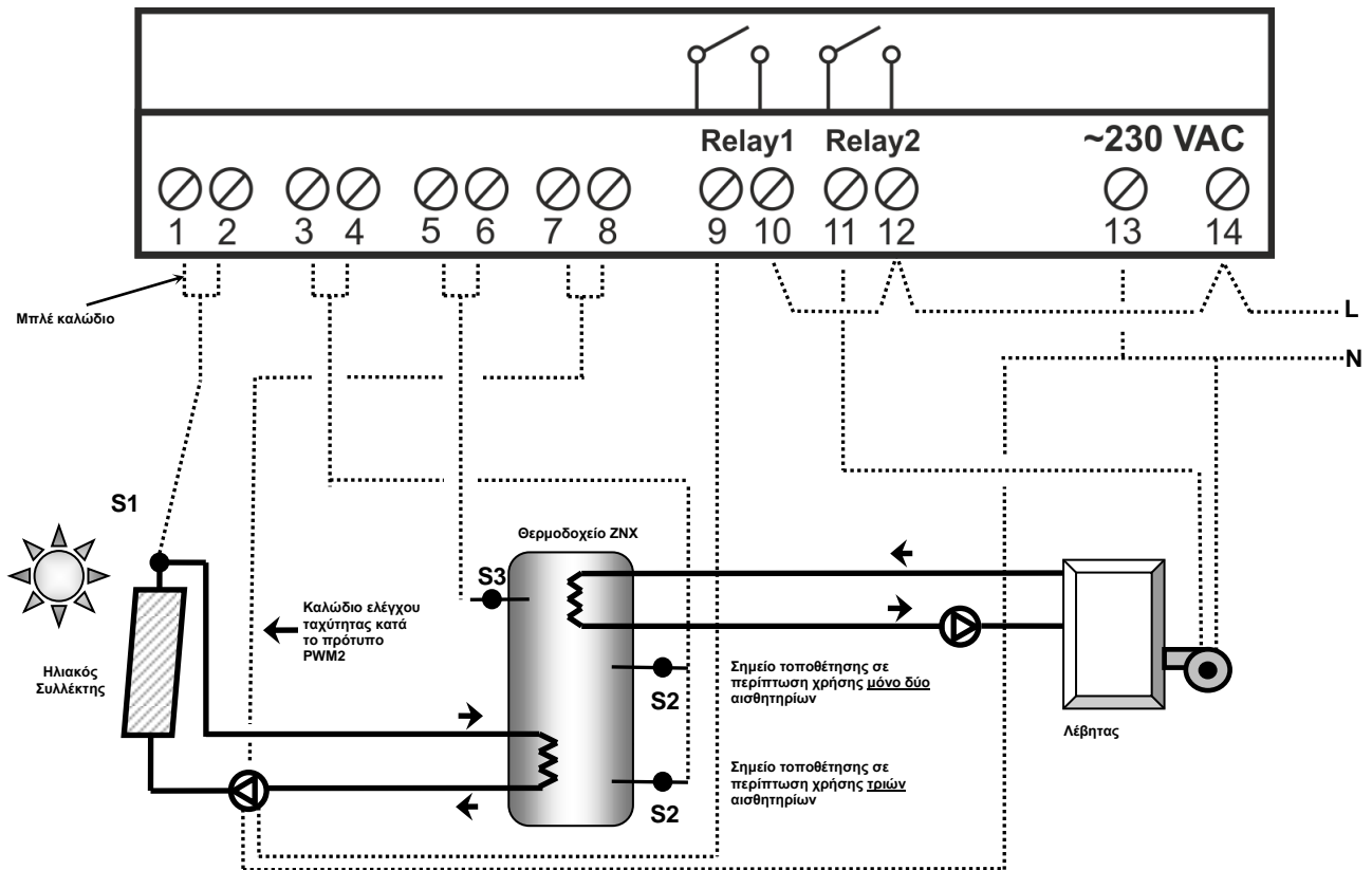
Σχήμα 1 Σχέδιο εγκατάστασης
