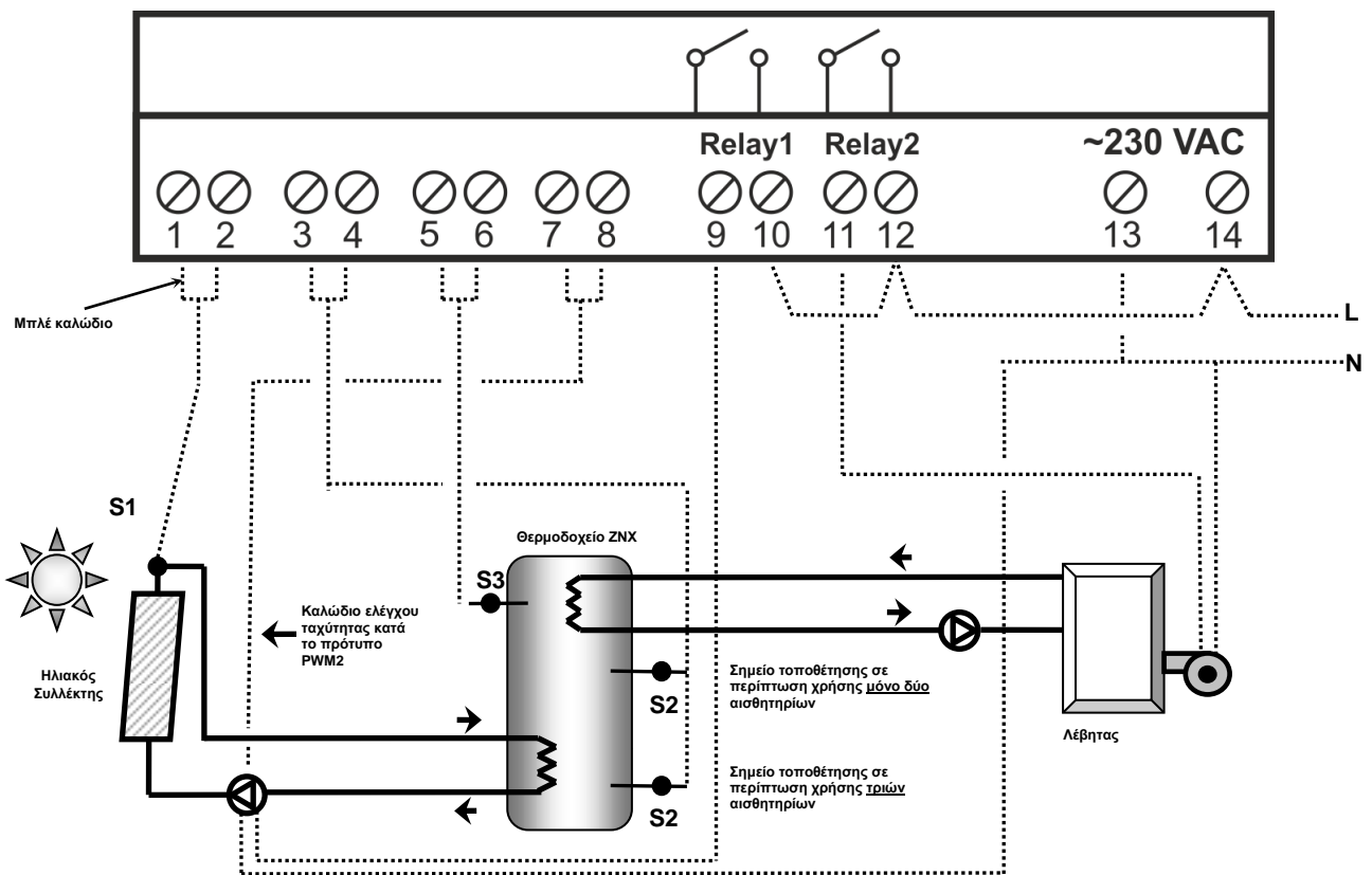
Σχήμα 1 Σχέδιο εγκατάστασης
