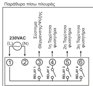
Εικόνα 1 Κλέμα ηλεκτρολογικής σύνδεσης
