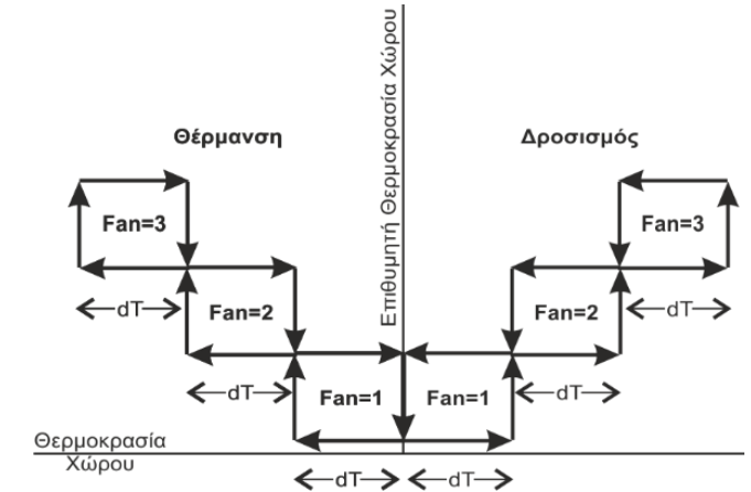
Εικόνα 2- Λειτουργία Αυτόματης Μετάπτωσης Ταχυτήτων
